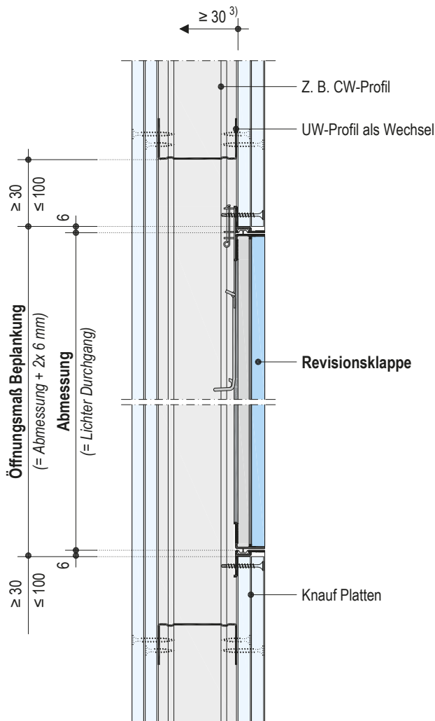
3) Bewegungsspielraum Revisionsklappe
