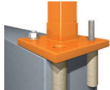
Verankerung in Beton gemäss ETAG N 001.
