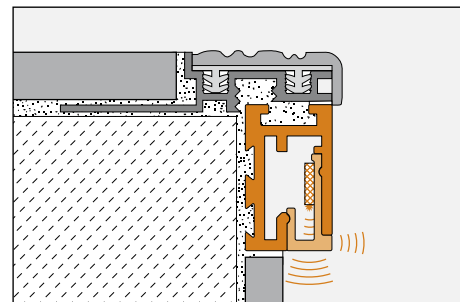
Einbaubeispiel mit Streuscheibe Schlüter®-LIPROTEC-PBD
