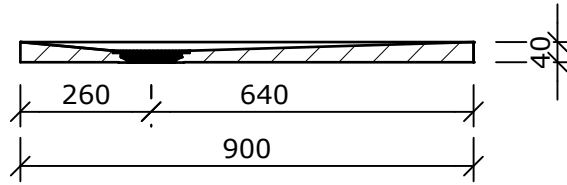
Schnitt A-A (1 : 15)
