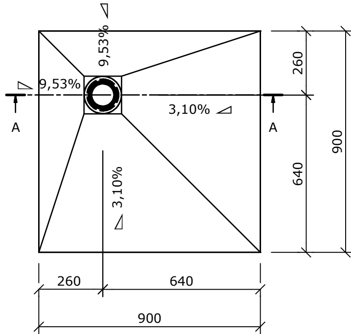
Draufsicht (1 : 15)
