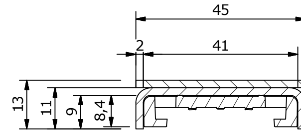
Schnitt B-B (1 : 1)
