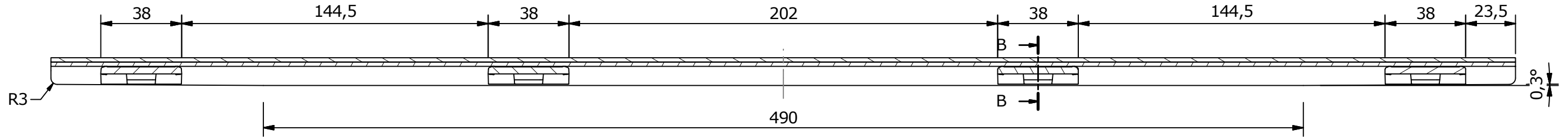
Schnitt A-A (1 : 2)
