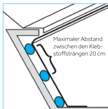
Beispiel: Lichtkuppelanschluss
